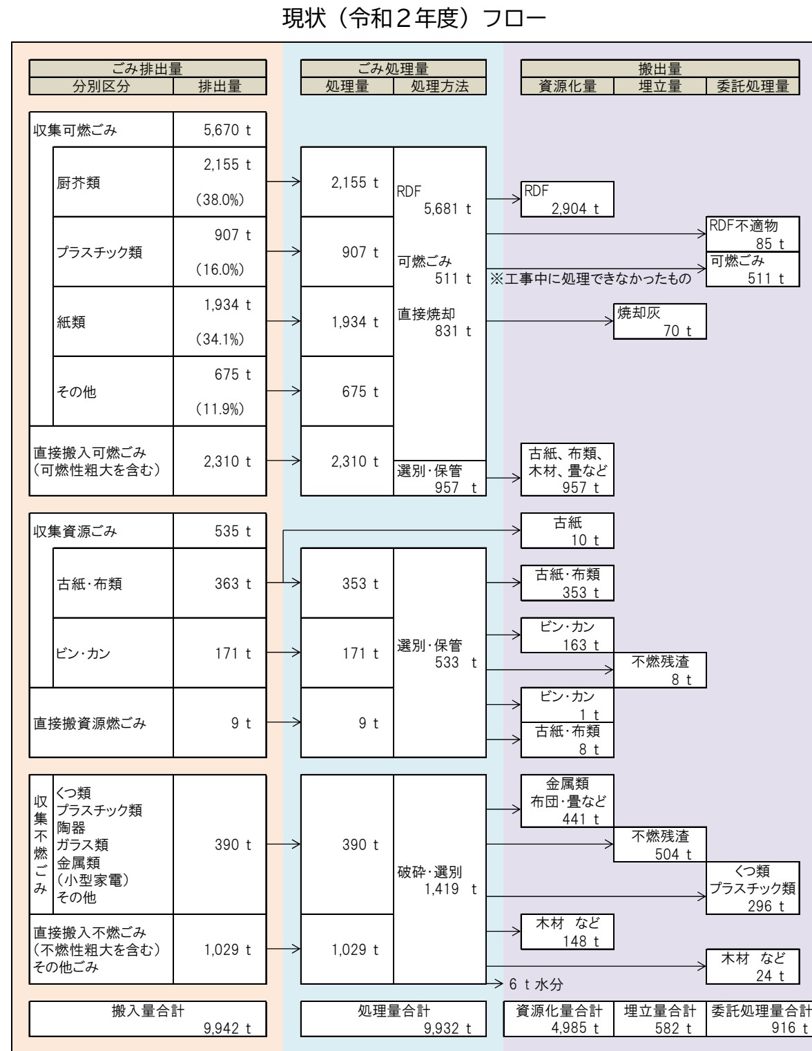
◆図表 19 (3) 雲南市の処理フロー
