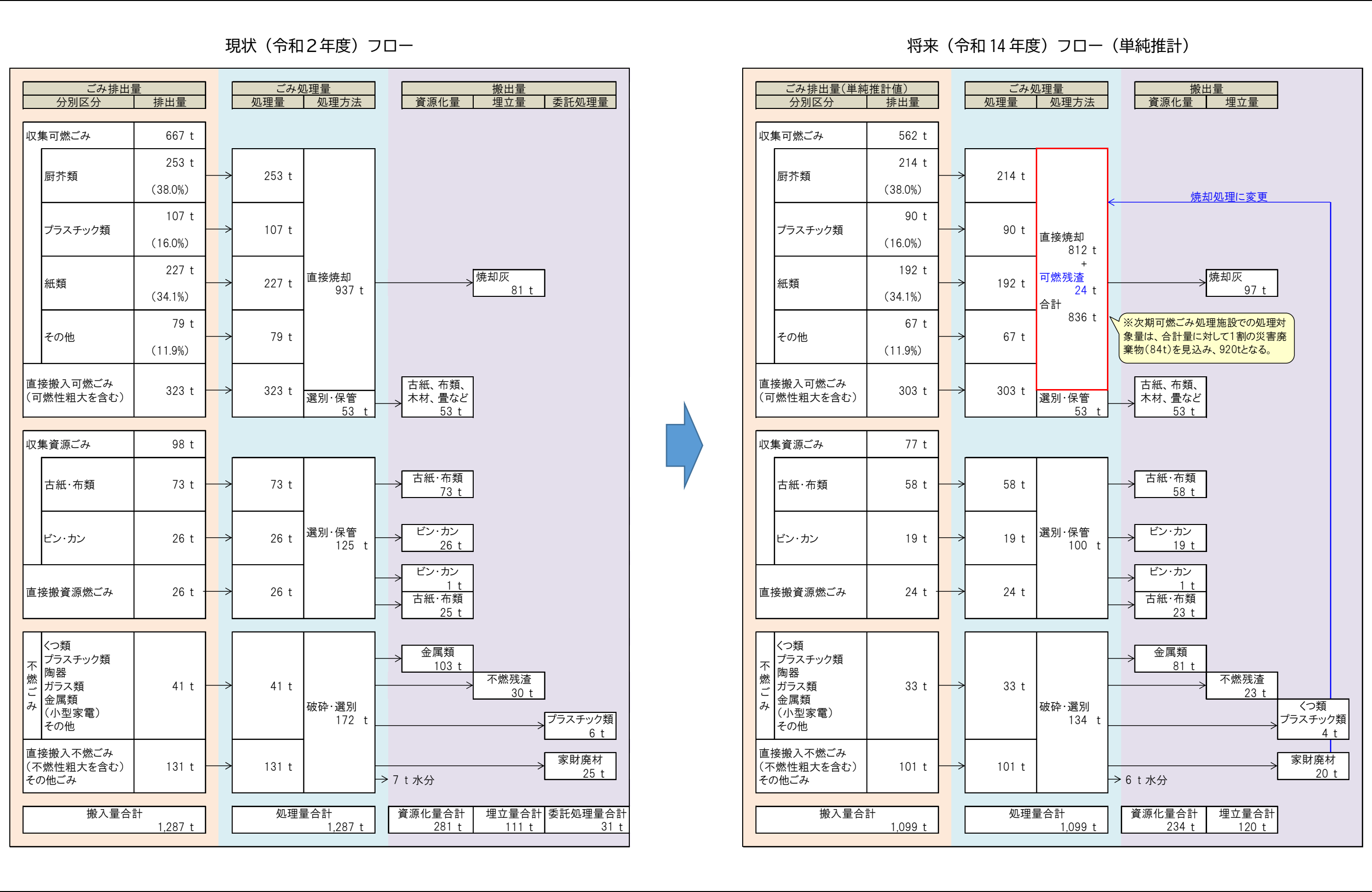
◆図表 20（1） 飯南町の処理フロー
