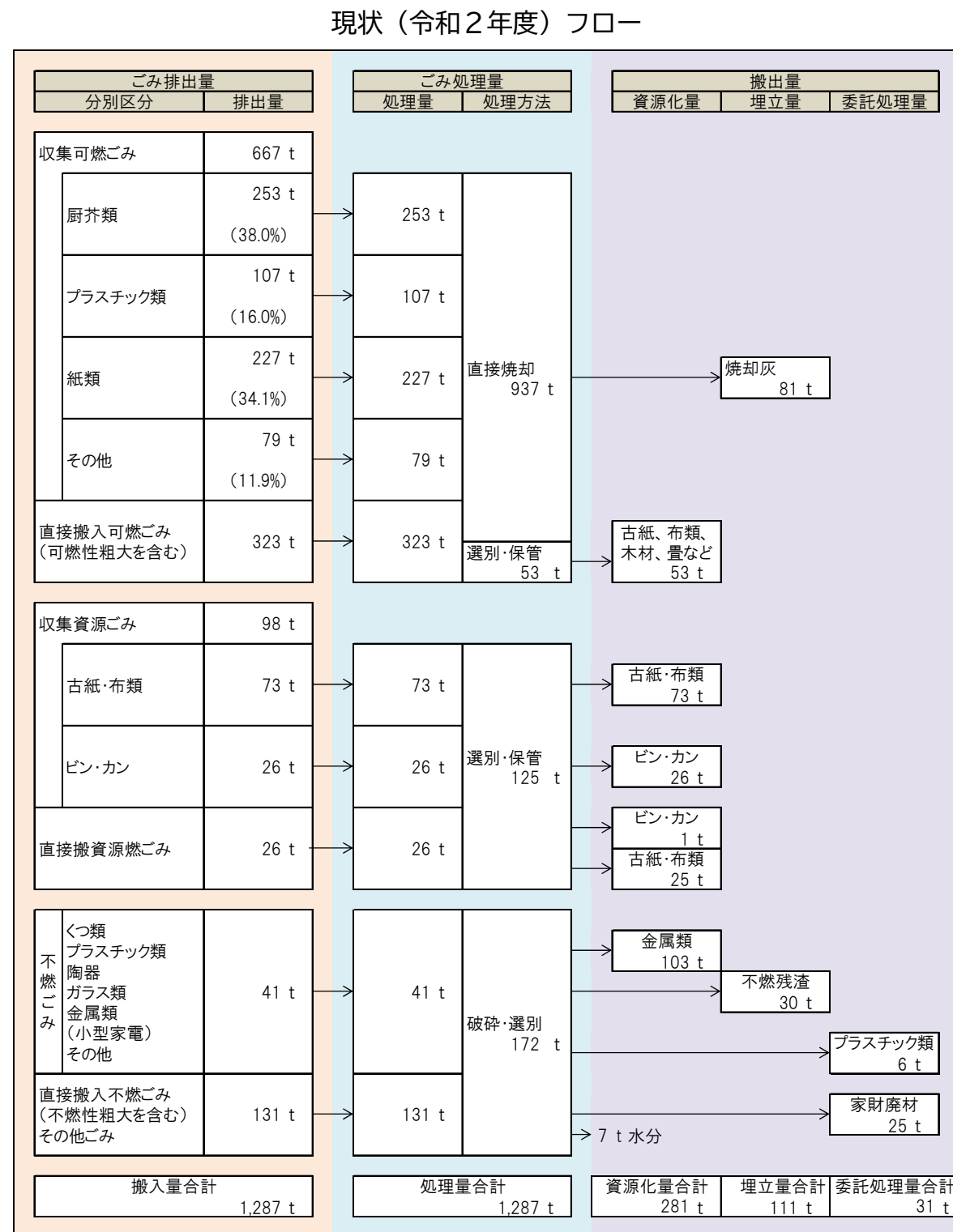
◆図表 20 (3) 飯南町の処理フロー
