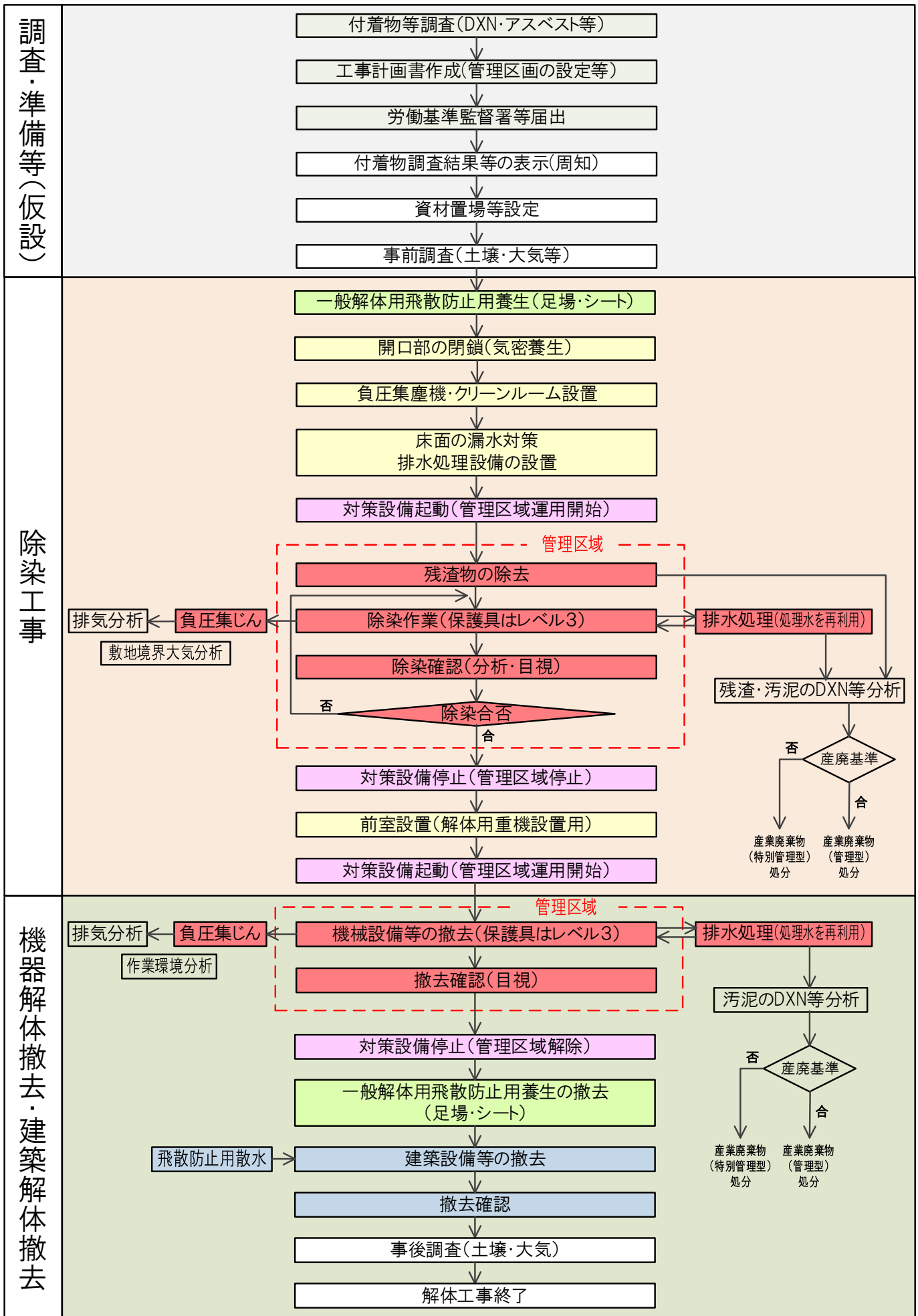
参考 一般的な焼却施設解体工事フロー図
